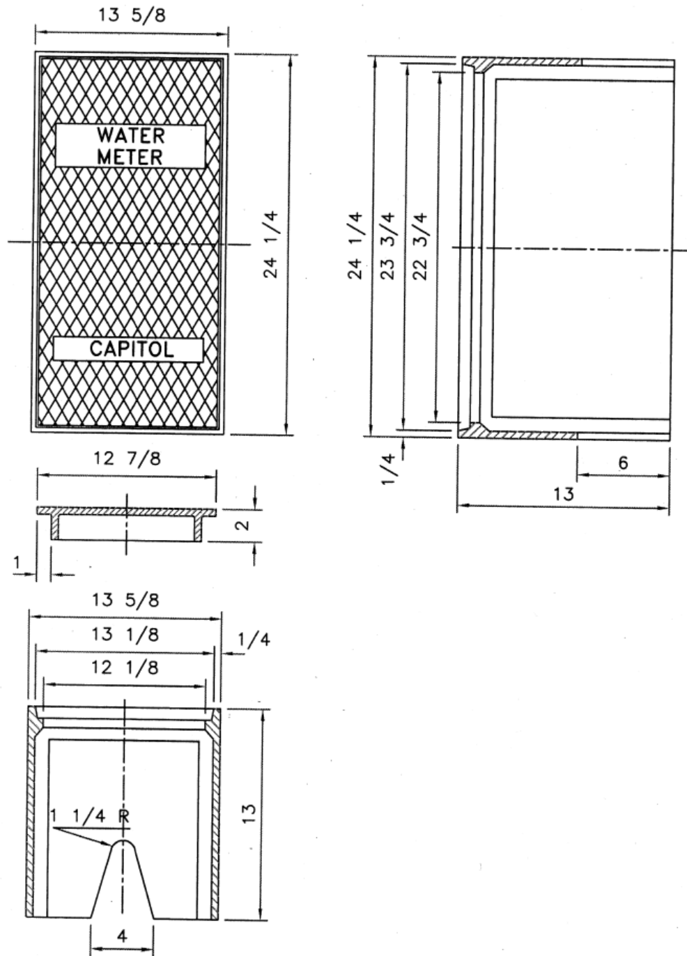
D-112 / MBX-3 METER BOX & LID
